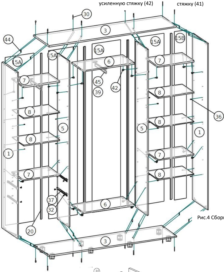
Рис.2 Схема сборки на эксцентриковую усиленную стяжку (42)
